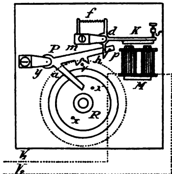
Č. 1737. Hippovy sekundární, elektrické hodiny.
